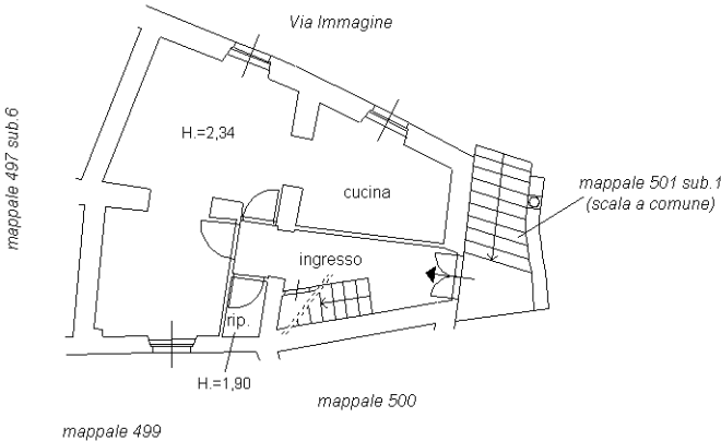
PIANO PRIMO
